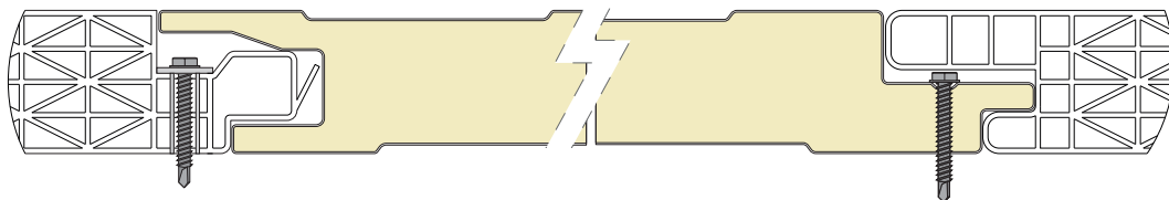
Detalle unión Panel PRAGA FACHADA de 35mm y DUBAI POLIFAM35.
