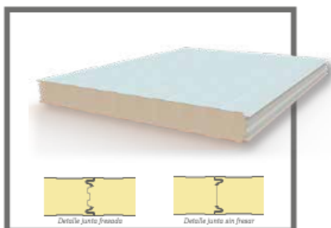
Imágenes del panel OSLO 1125 - PUR/PIR fijado. No es necesario incorporar junta
